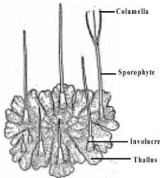
Figure12- Aspect des Anthocéroterées
