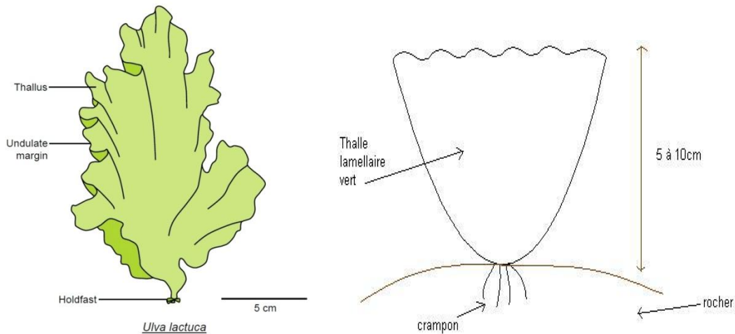
Figure 33- L'aspect du thalle d' Ulva lactuca
