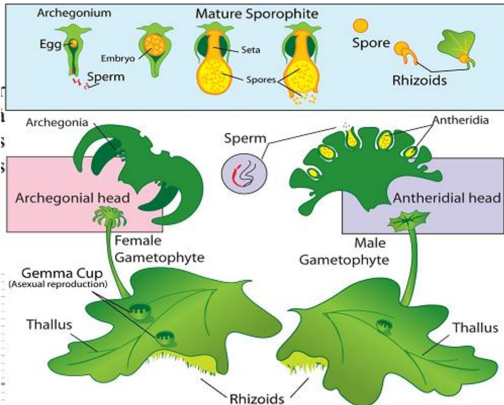
Figure11- Le cycle de vie des hépatiques
