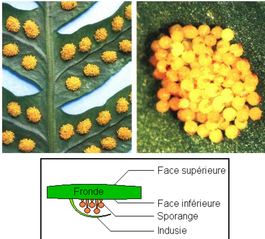
Figure3- Les sporanges d'une fougère.
