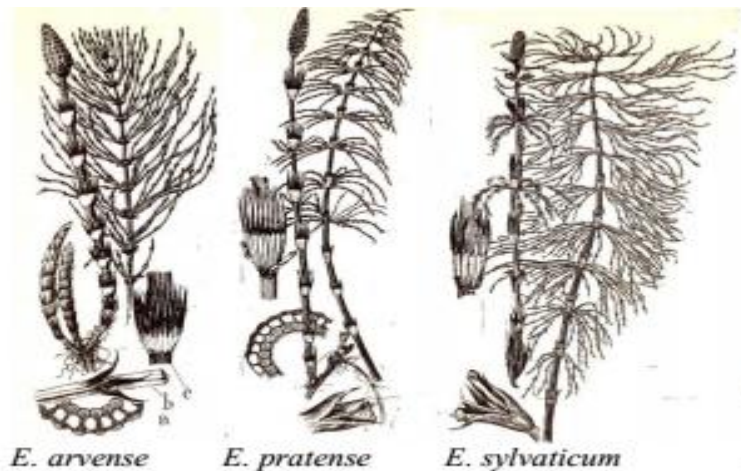
Figure8- Les Equisetinées ou prêles
