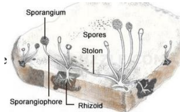
Figure14- Développement du Rhizopus sur le substrat (morceau de pain)
