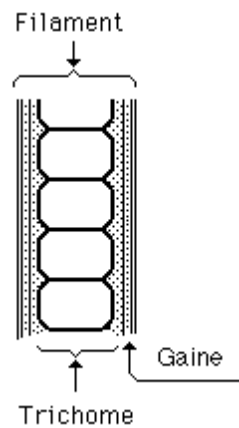
Figure3- Colonies et filaments des cyanobactéries
