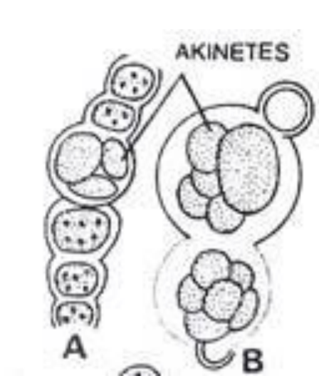
Figure 12- Germination des akinètes chez Nostoc
