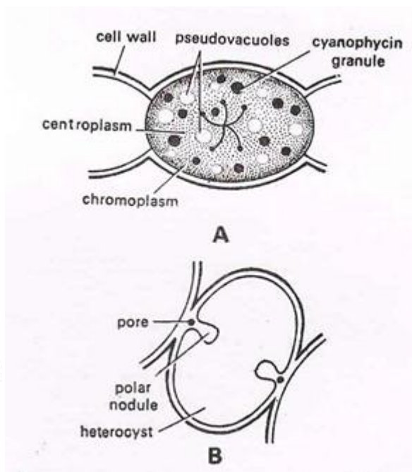
Figure 11- A. Cellule végétative de Nostoc B. Hétérocyste de Nostoc
