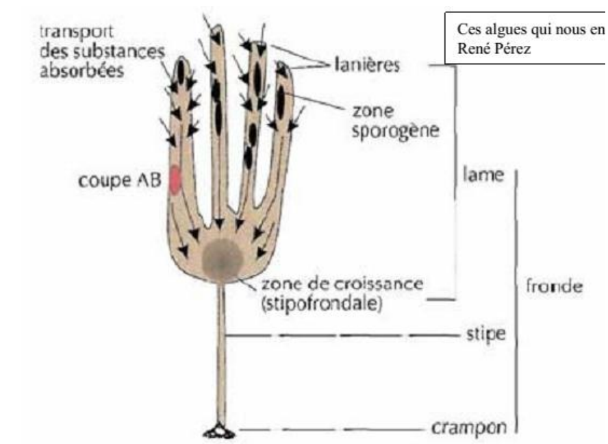
Figure15- Organisation du thalle de Laminaria digitata
