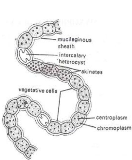
Figure 10- Un filament de Nostoc
